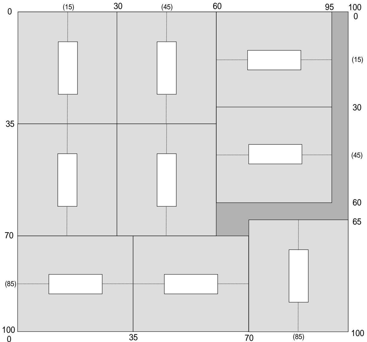
緊結タイプ用ゴム板割付 (100mm × 100mm; 厚み5mm)
